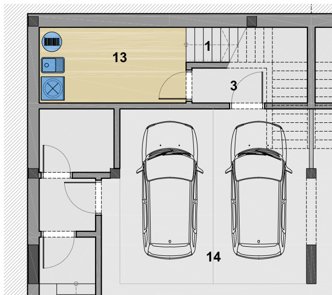
PLANTA SOTERRANI
