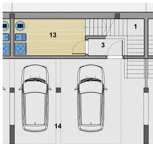
PLANTA SOTERRANI
