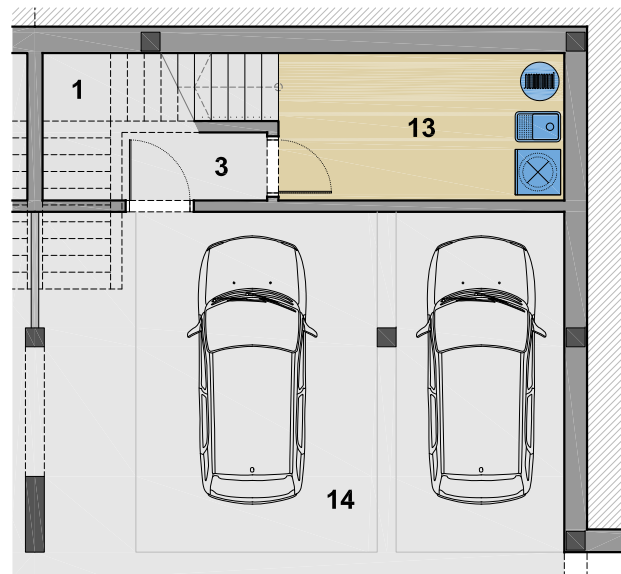
PLANTA SOTERRANI
