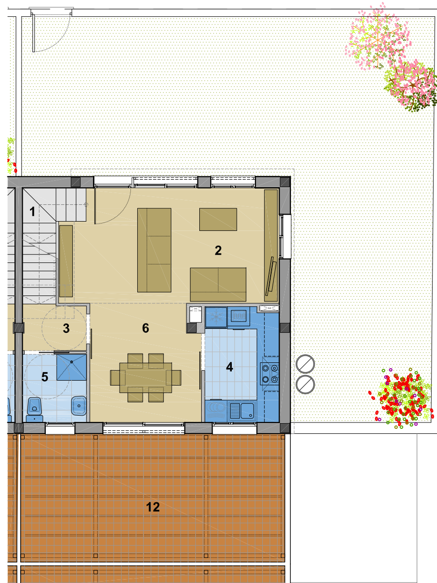
PLANTA BAIXA
