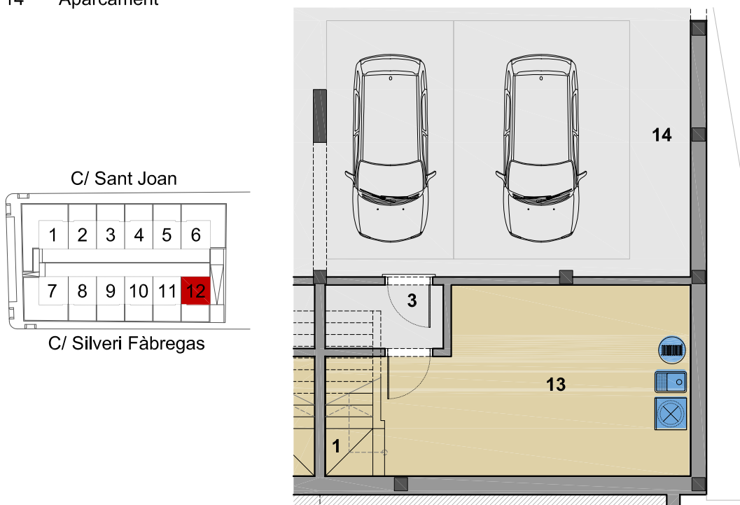
PLANTA SOTERRANI
